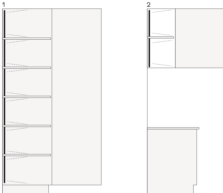
1 Colonne con lampade verticali multiled, h da 1320 fino a 2280 2 Pensili con lampade verticali multiled, h da 360 fino a 1200
