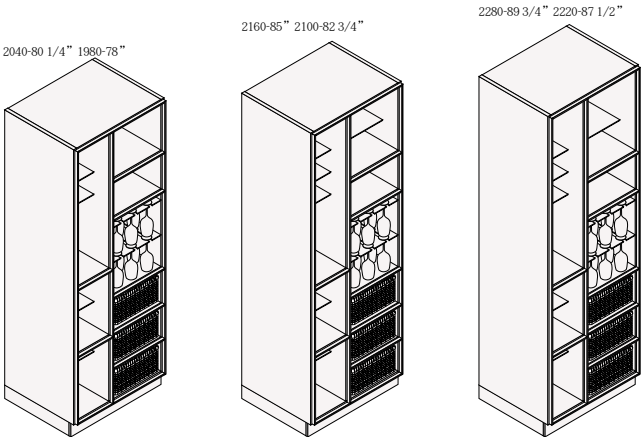
Colonna sinistra l 750 p 570
