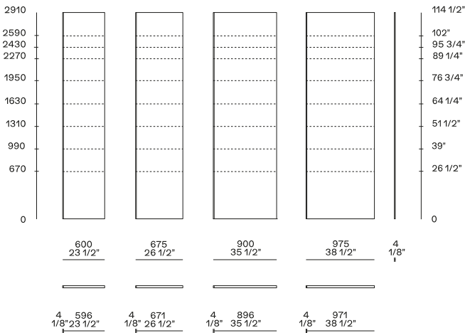
Inalco MDi® h max 1950 护壁板 左侧型材面板宽度为4 毫米
