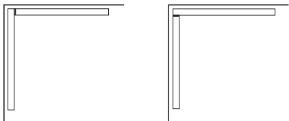
内角，在回扣面板上配置标准型材。
