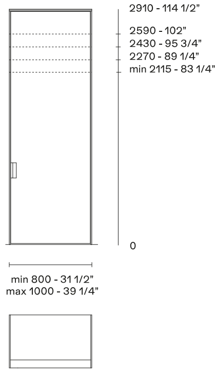
Puerta sencilla
