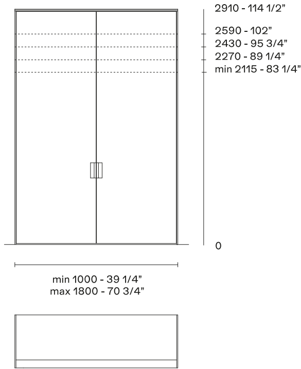
Puerta doble
